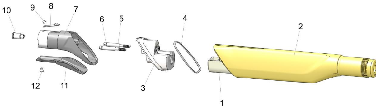
OptiGun GA03-P – shaft
