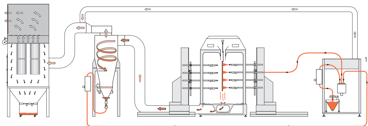
'OptiCenter dotato di cono per sacchetti di polvere fresca
